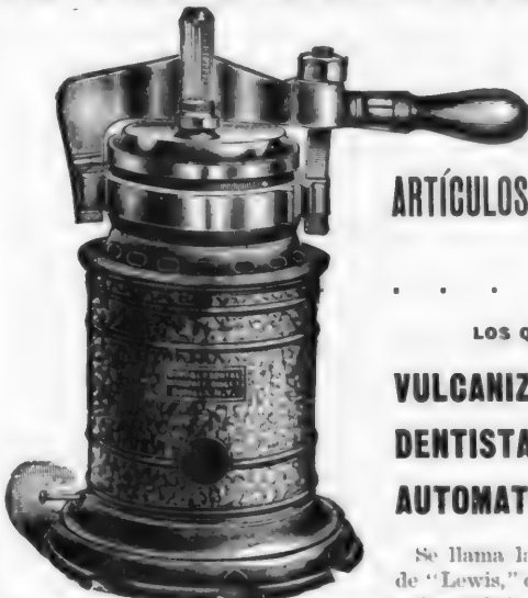
El Vulcanizador de "Lewis" con palanca atravesada y aparato para calentar con gas. Patentado el 2 de octubre de 1894.
